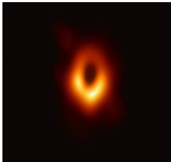
Figura 2: Primera imagen de un agujero negro situado en el centro de la galaxia M87, obtenida utilizando el Event Horizon Telescope. Foto tomada de www.eventhorizontelescope.org . Créditos: Event Horizon Telescope Collaboration
